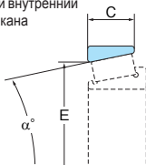
Рис. 1. Размеры субблока
