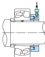
Рис. 8.45 Гидравлическая гайка
