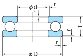
Рис 4.3 Одинарные упорные шариковые подшипники
